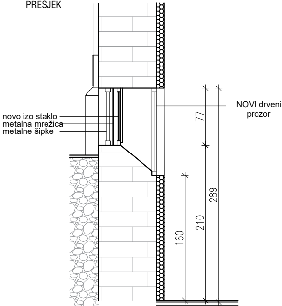
PRESJEK
