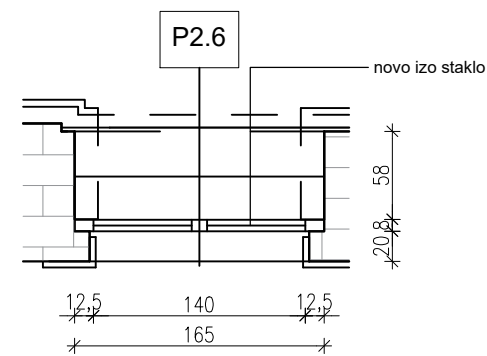
POGLED
