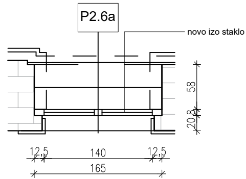
POGLED
