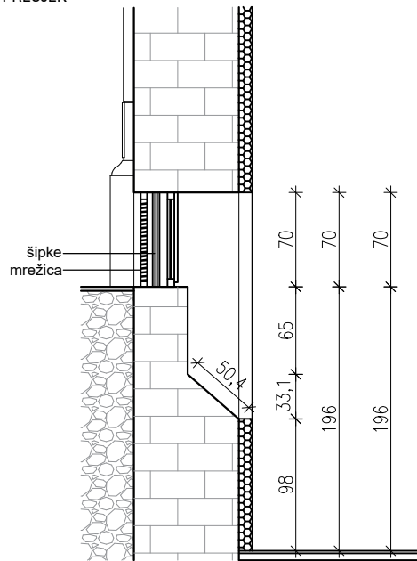
PRESJEK
