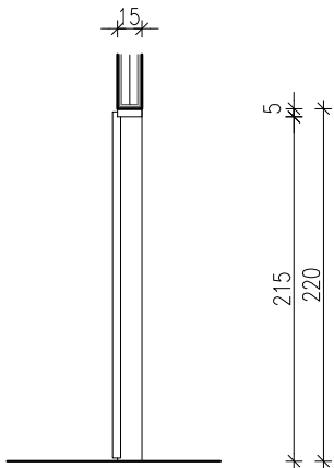
PRESJEK
