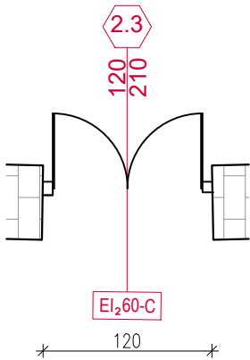
TLOCRT
