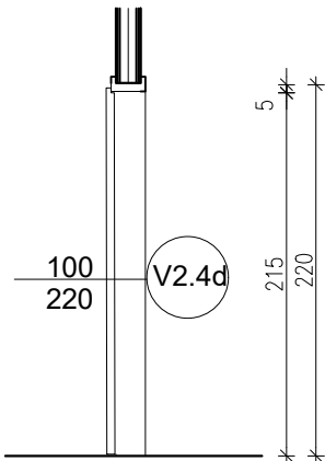
PRESJEK
