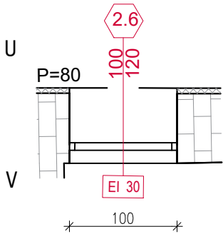
TLOCRT
