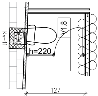
TLOCRT
