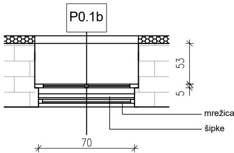
POGLED
