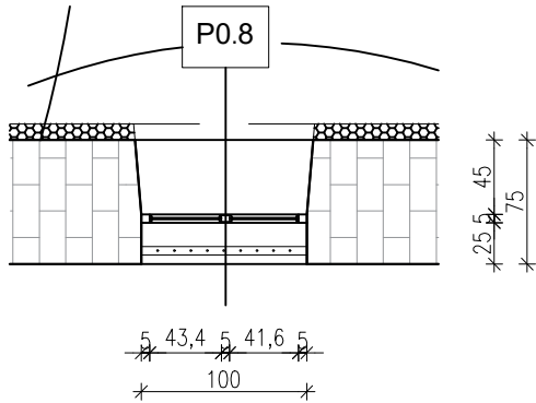
TLOCRT
