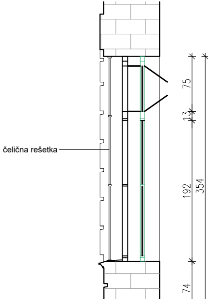
PRESJEK
