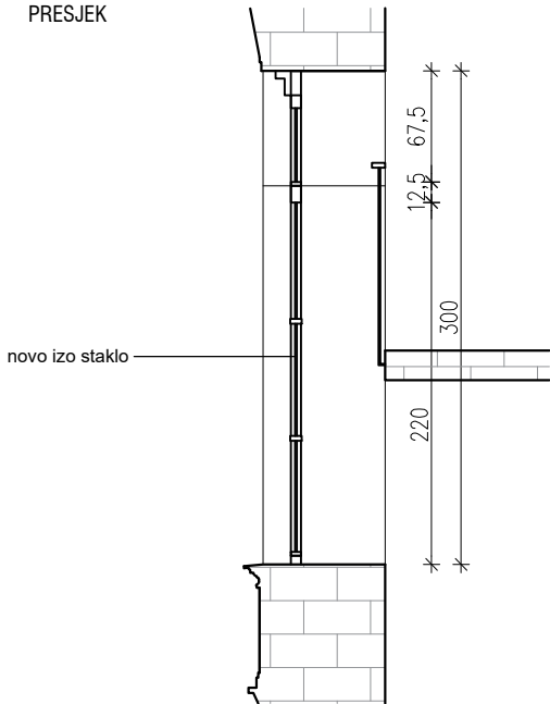
PRESJEK
