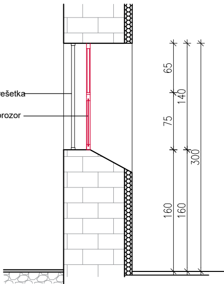
PRESJEK
