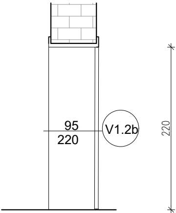
PRESJEK
