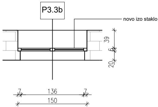
POGLED
