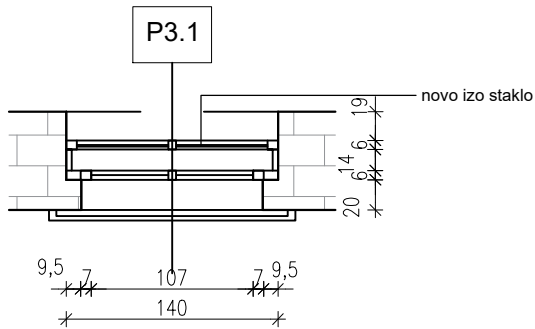
POGLED
