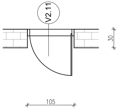
TLOCRT
