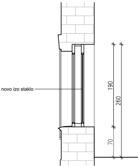
PRESJEK
