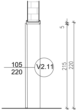
PRESJEK
