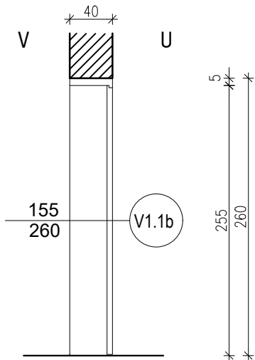
PRESJEK
