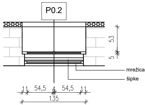
TLOCRT
