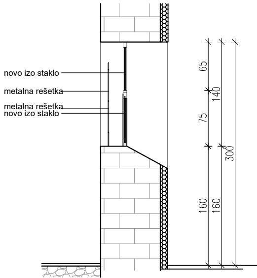
PRESJEK
