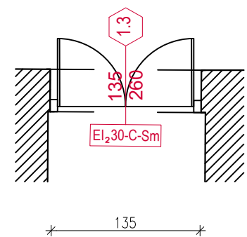
POGLED
