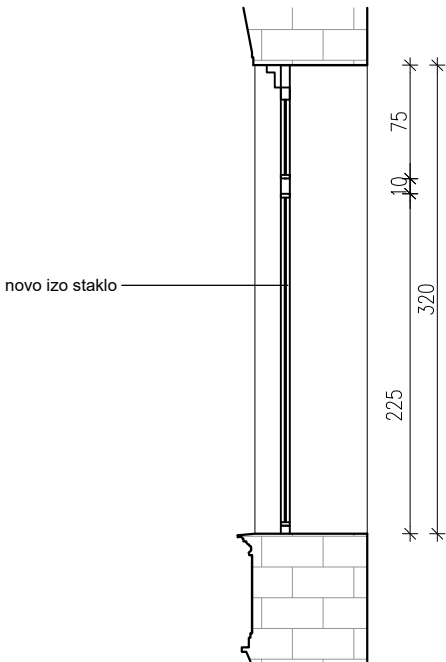
PRESJEK
