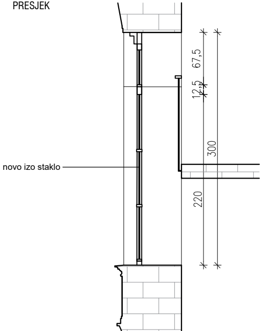
PRESJEK
