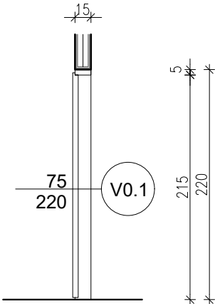
PRESJEK
