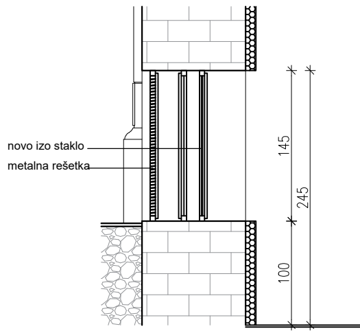
PRESJEK
