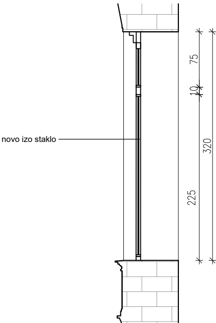
PRESJEK
