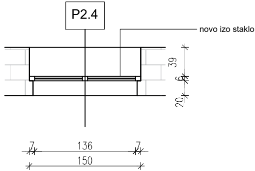
POGLED
