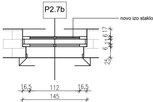
POGLED
