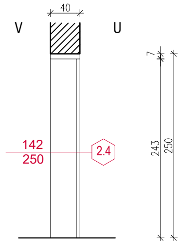
PRESJEK
