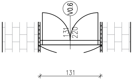
TLOCRT
